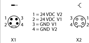
Alimentation en tension 7/8"
