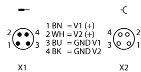
Alimentation en tension M8 × 1
