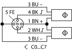
M12 x 1输入接口
