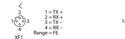
EtherCAT
